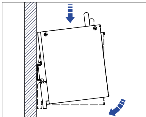
Abb. 3: Installation des Gateways auf Normschiene
