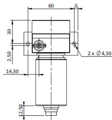
Connectique C (connecteur M16 - DIN 8 broches)
