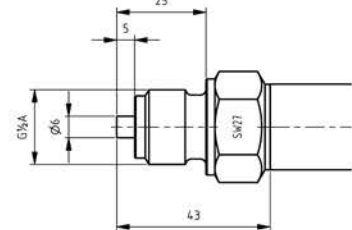
Fig. 6 - G 1/2 M, Manomètre EN837
